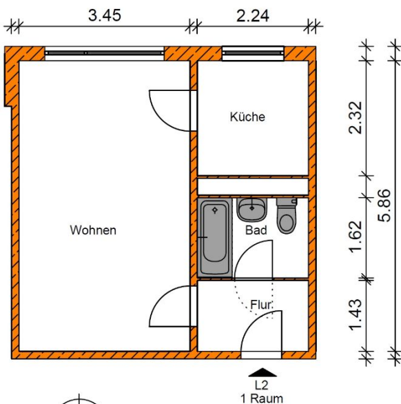
Wohn-/Schlafzimmer
